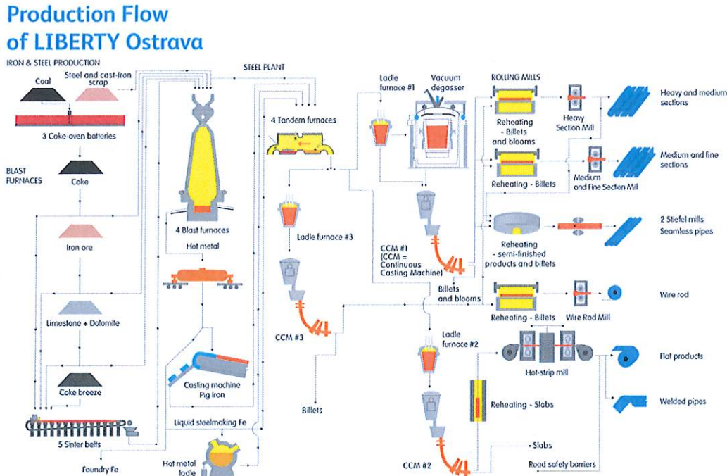
Obr. 1: Schéma výrobního procesu
