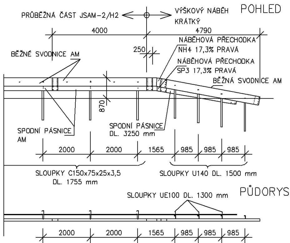
Obrázek 36 – Krátký výškový náběh svodidla JSAM-2/H2
