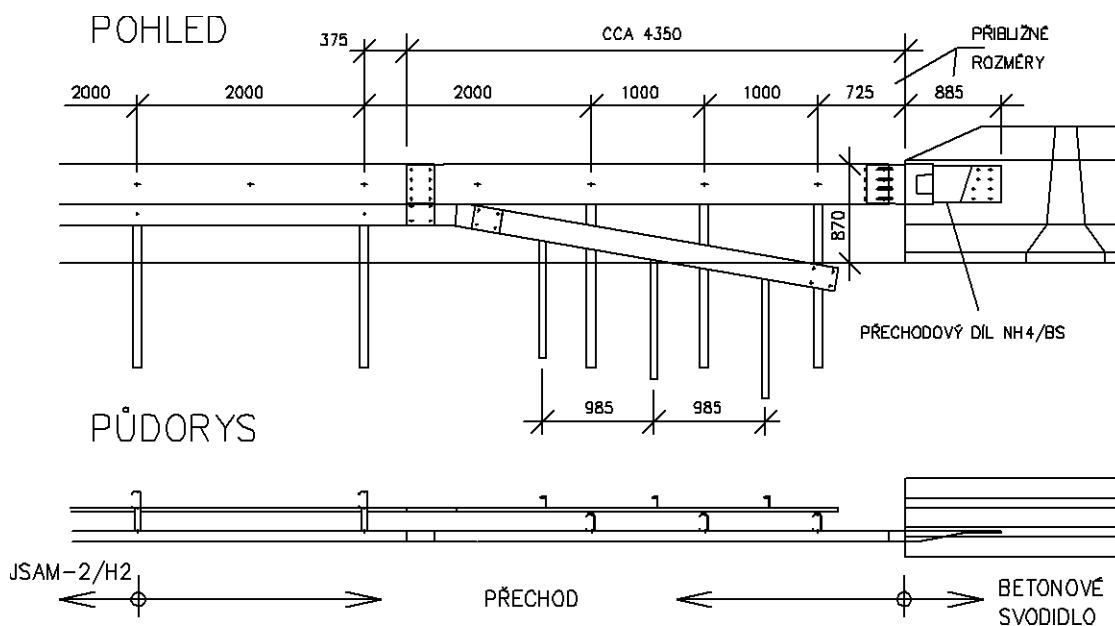
Obrázek 74 - Přejchod z JSAM-2/H2 na betonové svodidlo
