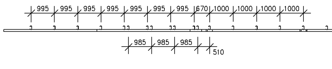
Obrázek 47 – Výškový náběh svodidla JSA-AM-1/H2
