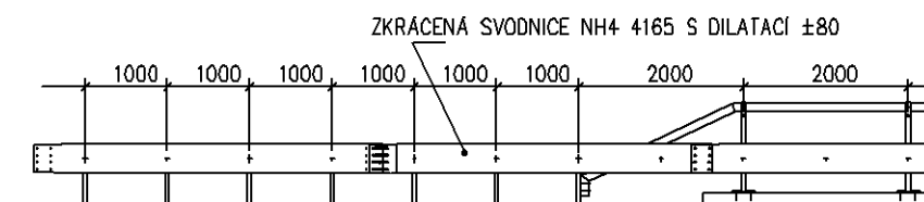
Obrázek 65 – Příklad dilatace před mostem
