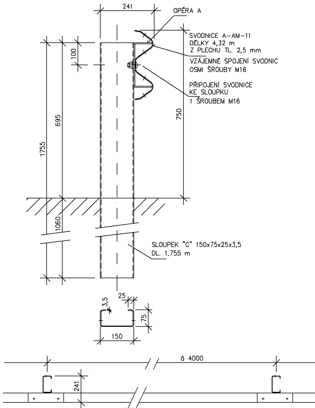
Obrázek 18 - Svodidlo JSA-AM-4/H1
