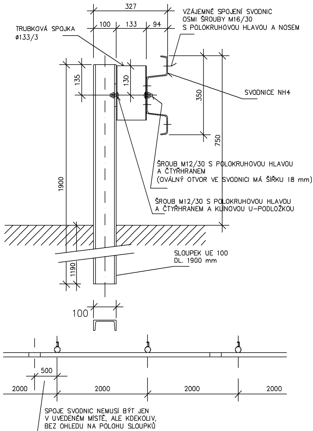
Obrázek 2 - Svodidlo JSNH4/H1
