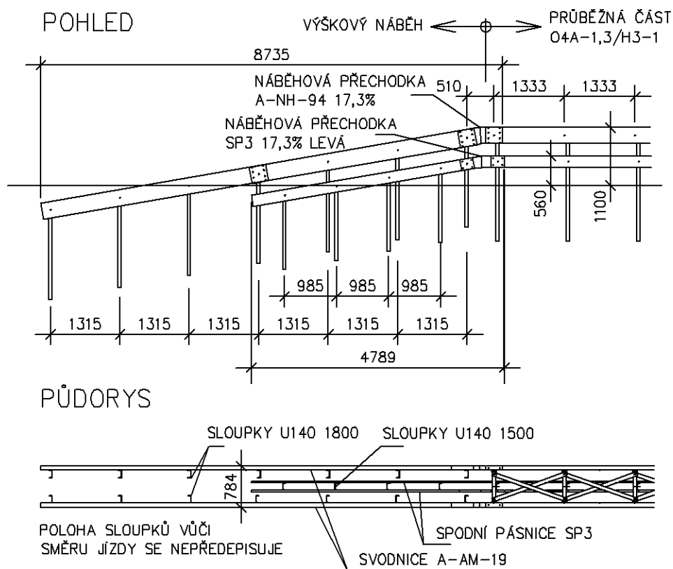
Obrázek 53 – Výškový náběh svodidla O4A-1,3/H3-1
