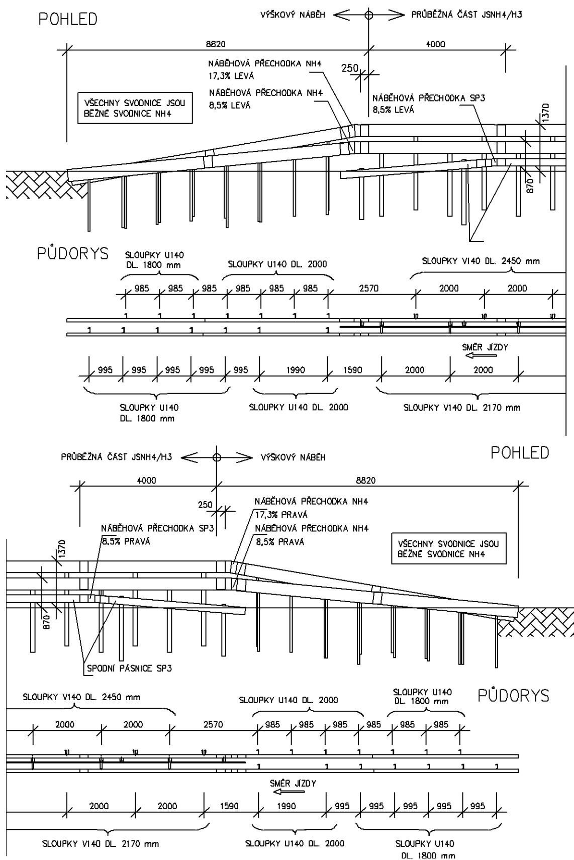
Obrázek 26 – Výškový náběh svodidla JSNH4/H3 (svodidlo má jen jeden náběh)
