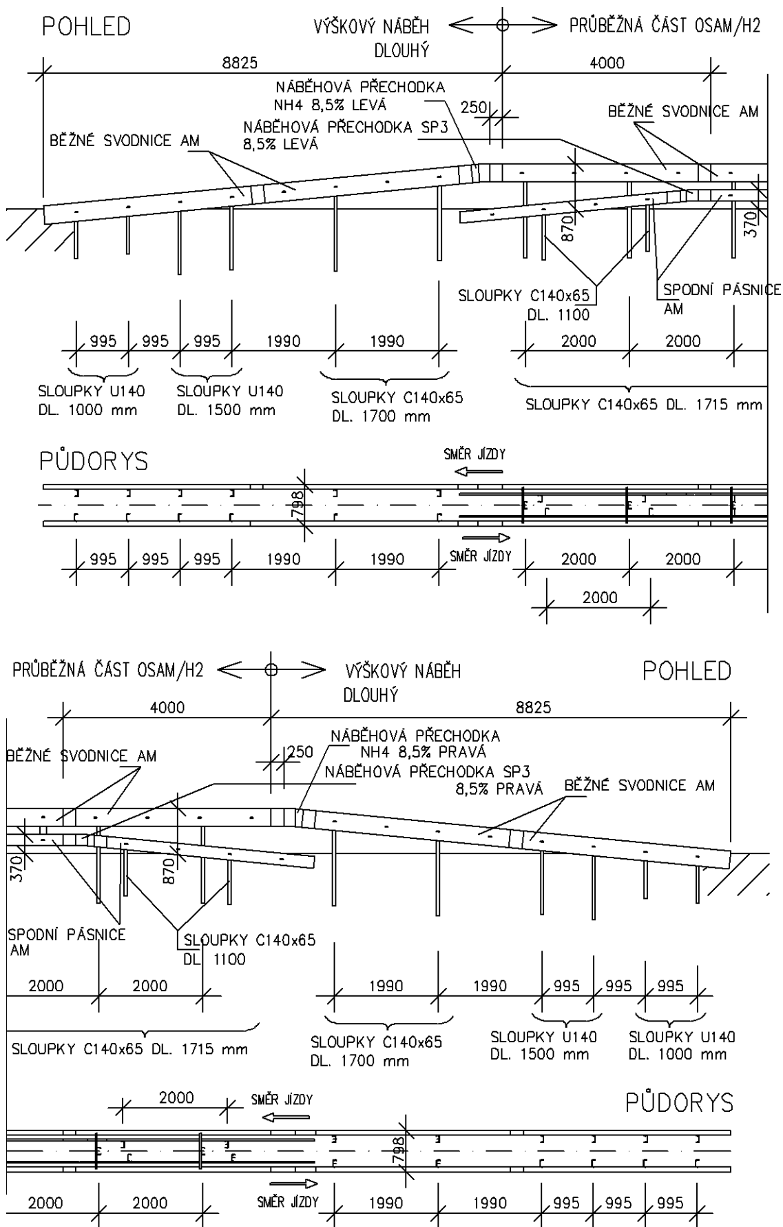
Obrázek 39 – Dlouhý výškový náběh svodidla OSAM/H2
