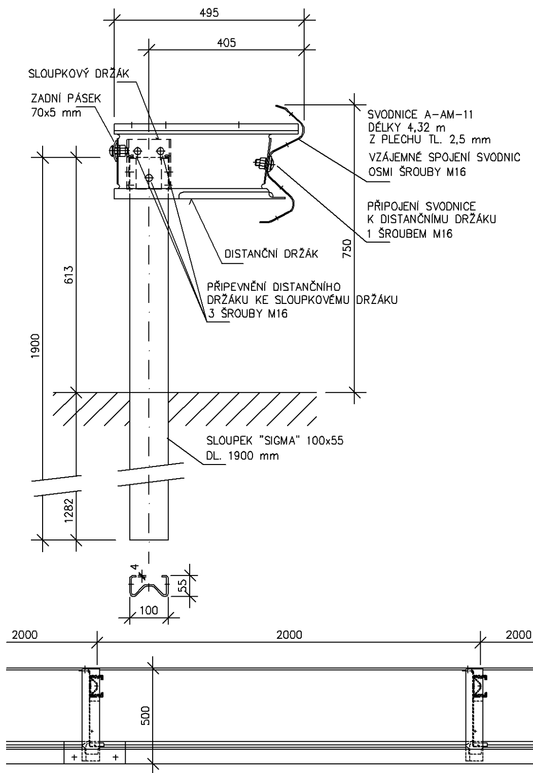
Obrázek 17 - Svodidlo JSA-AM-2/H1
