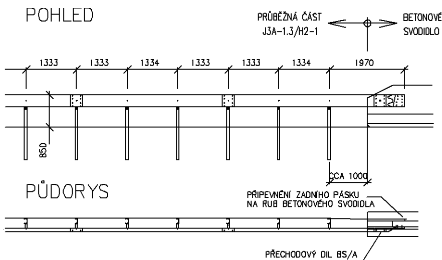
Obrázek 78 – Přejchod J3A-1,3/H2-1 na betonové svodidlo
