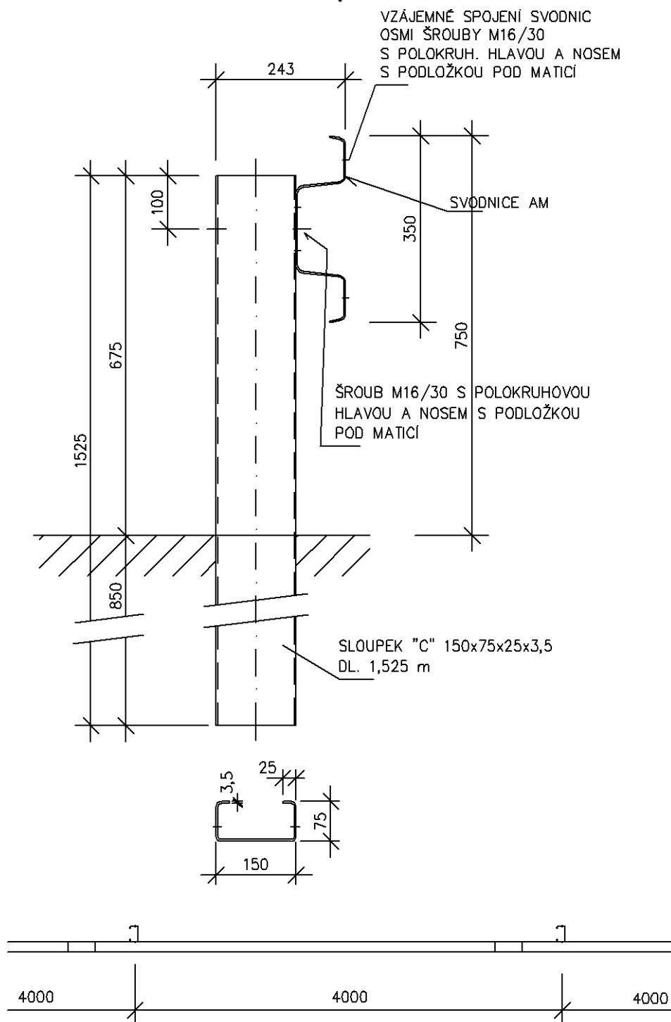
Obrázek 9 - Svodidlo JSAM-4/N2
