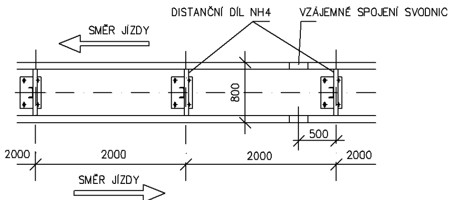
Obrázek 8 - Svodidlo OSPNH4/H3
