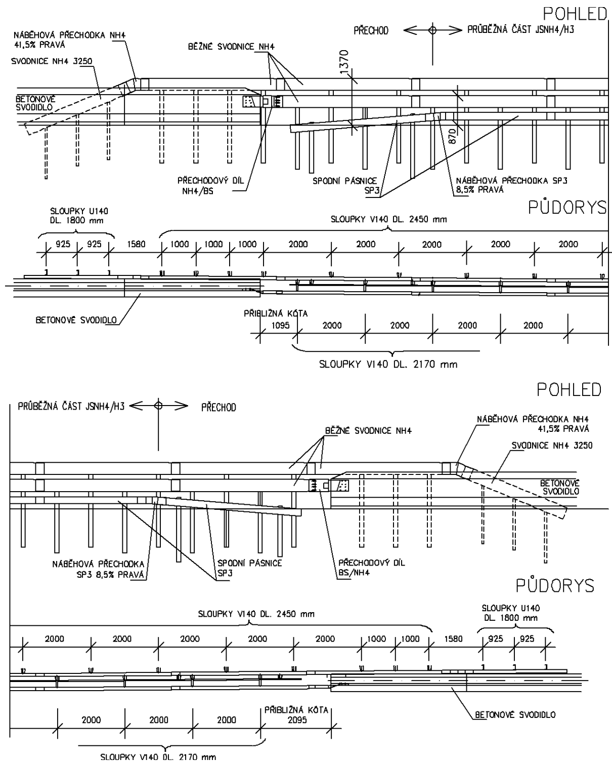
Obrázek 76 – Přechod JSNH4/H3 na betonové svodidlo
