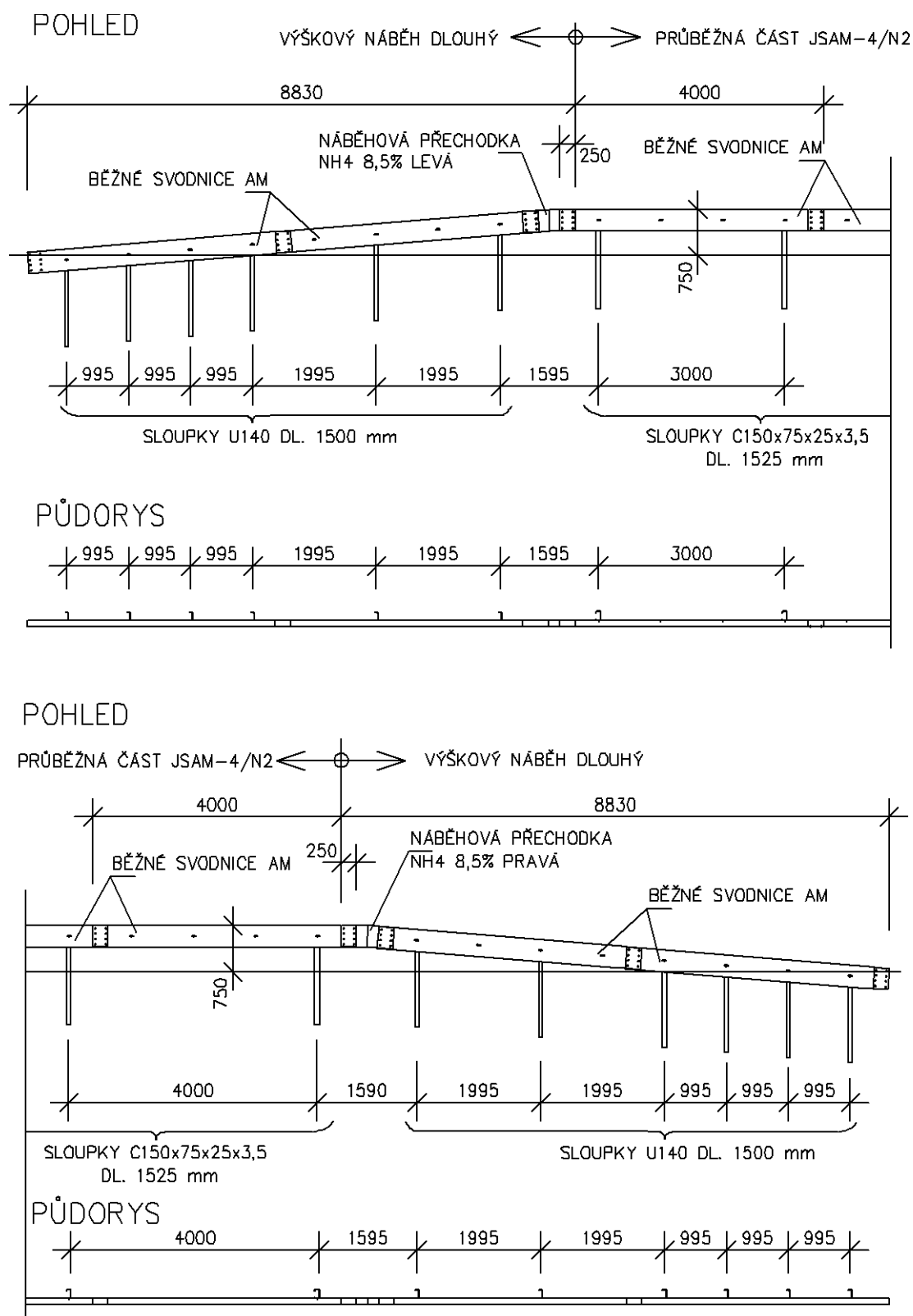
Obrázek 29 – Dlouhý výškový náběh svodidla JSAM-4/N2
