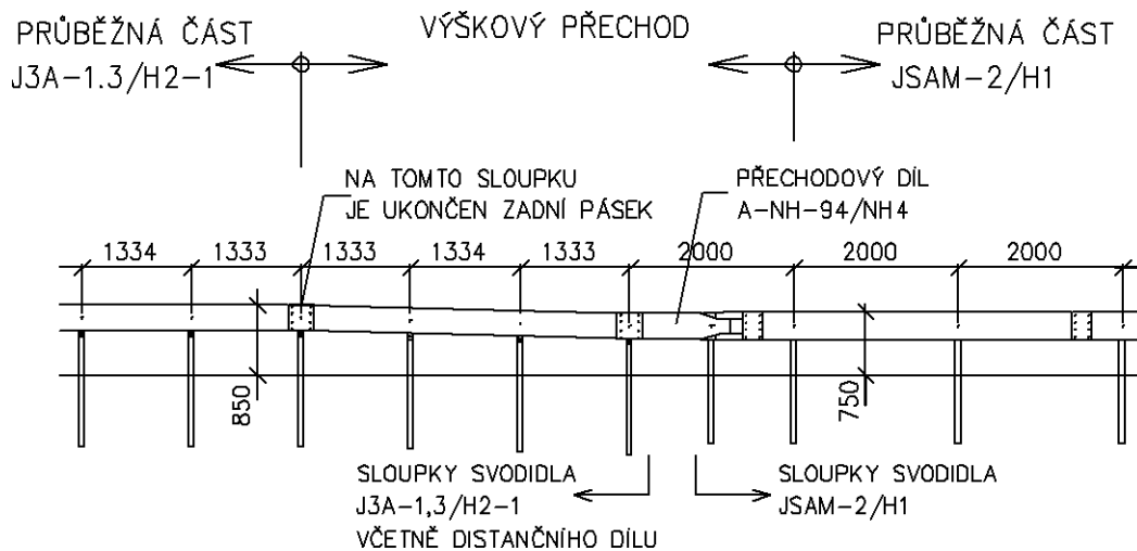
Obrázek 58 - Přejed z J3A-1,3/H2-1 na JSAM-2/H1
