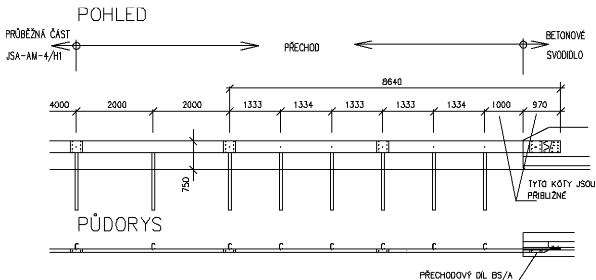
Obrázek 77 – Přejchod JSA-AM-4/H1 na betonové svodidlo
