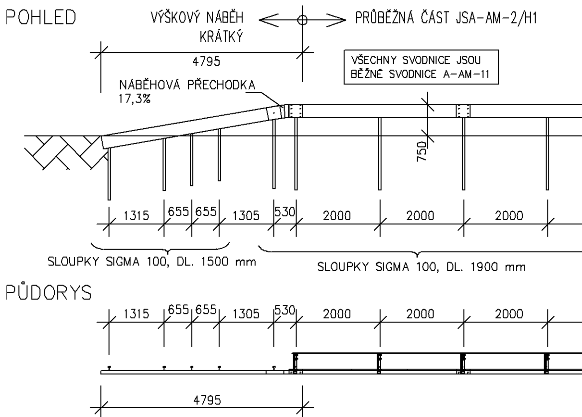
Obrázek 44 – Krátký výškový náběh svodidla JSA-AM-2/H1
