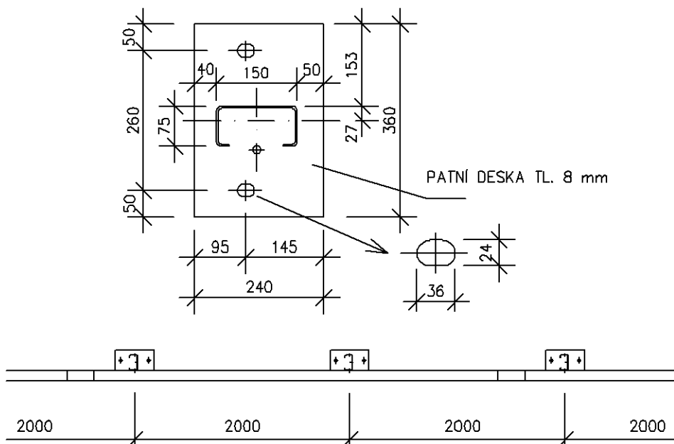
Obrázek 11 - Svodidlo JSPAM-2/H1
