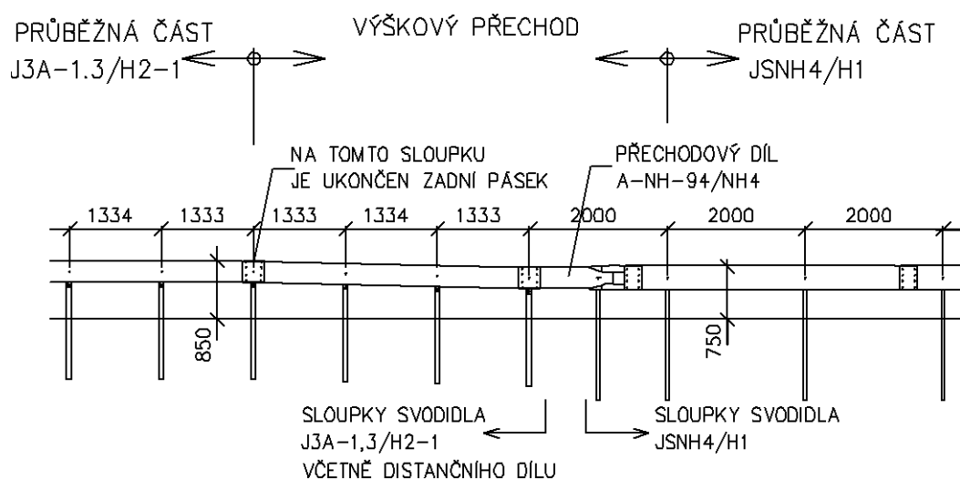
Obrázek 60 - Přejchod z J3A-1,3/H2-1 na JSN4/H1
