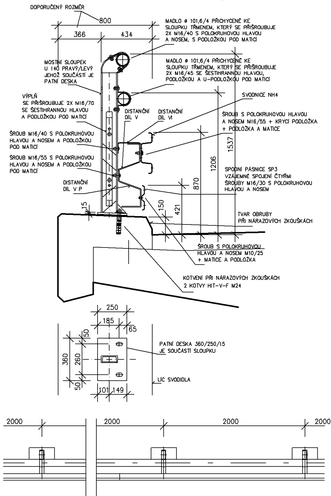
Obrázek 7 - Svodidlo ZSNH4/H3
