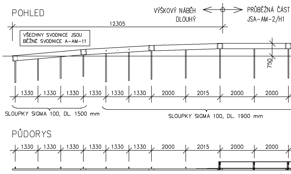
Obrázek 43 – Dlouhý výškový náběh svodidla JSA-AM-2/H1
