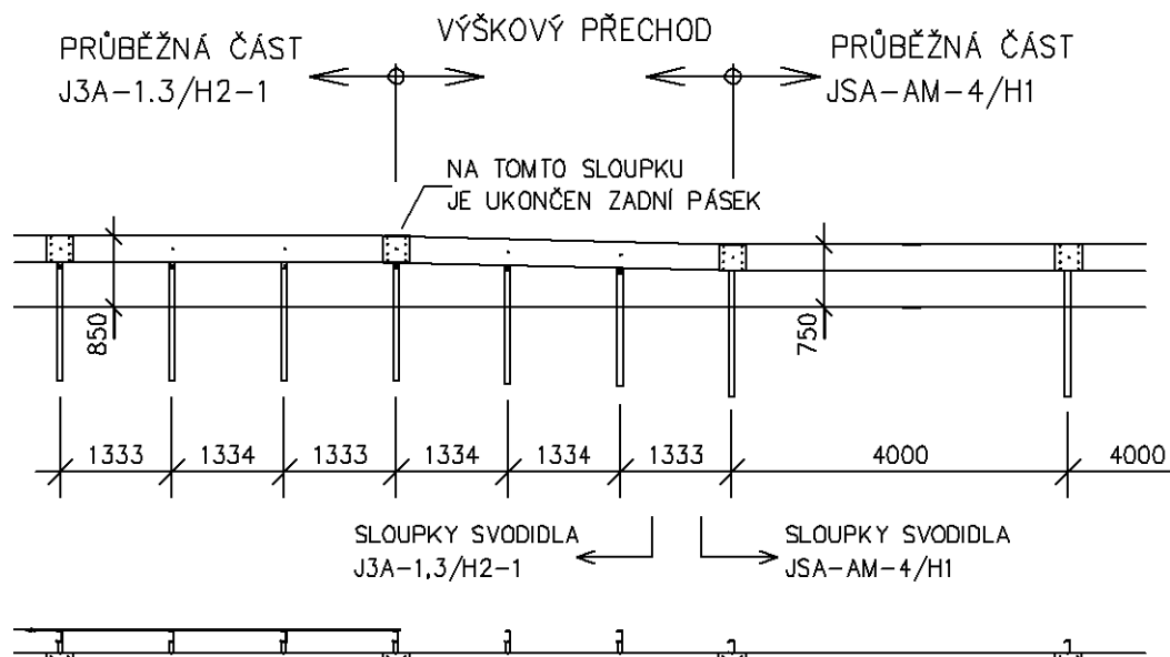
Obrázek 59 - Přejchod z J3A-1,3/H2-1 na JSA-AM-4/H1
