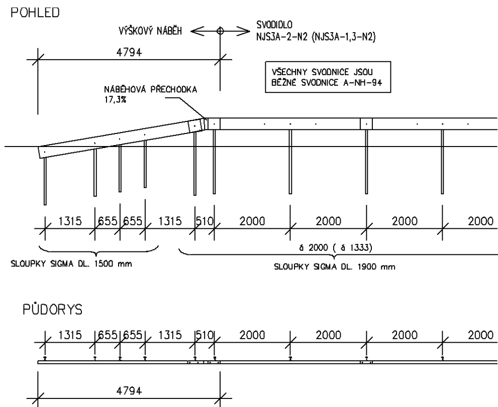
Obrázek 42 – Krátký výškový náběh svodidla NJS3A-2/N2 a NJS3A-1,3/N2
