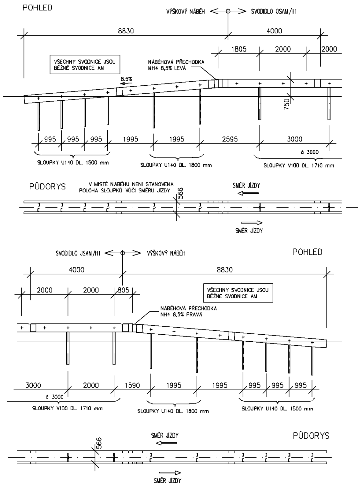
Obrázek 37 – Dlouhý výškový náběh svodidla OSAM/H1
