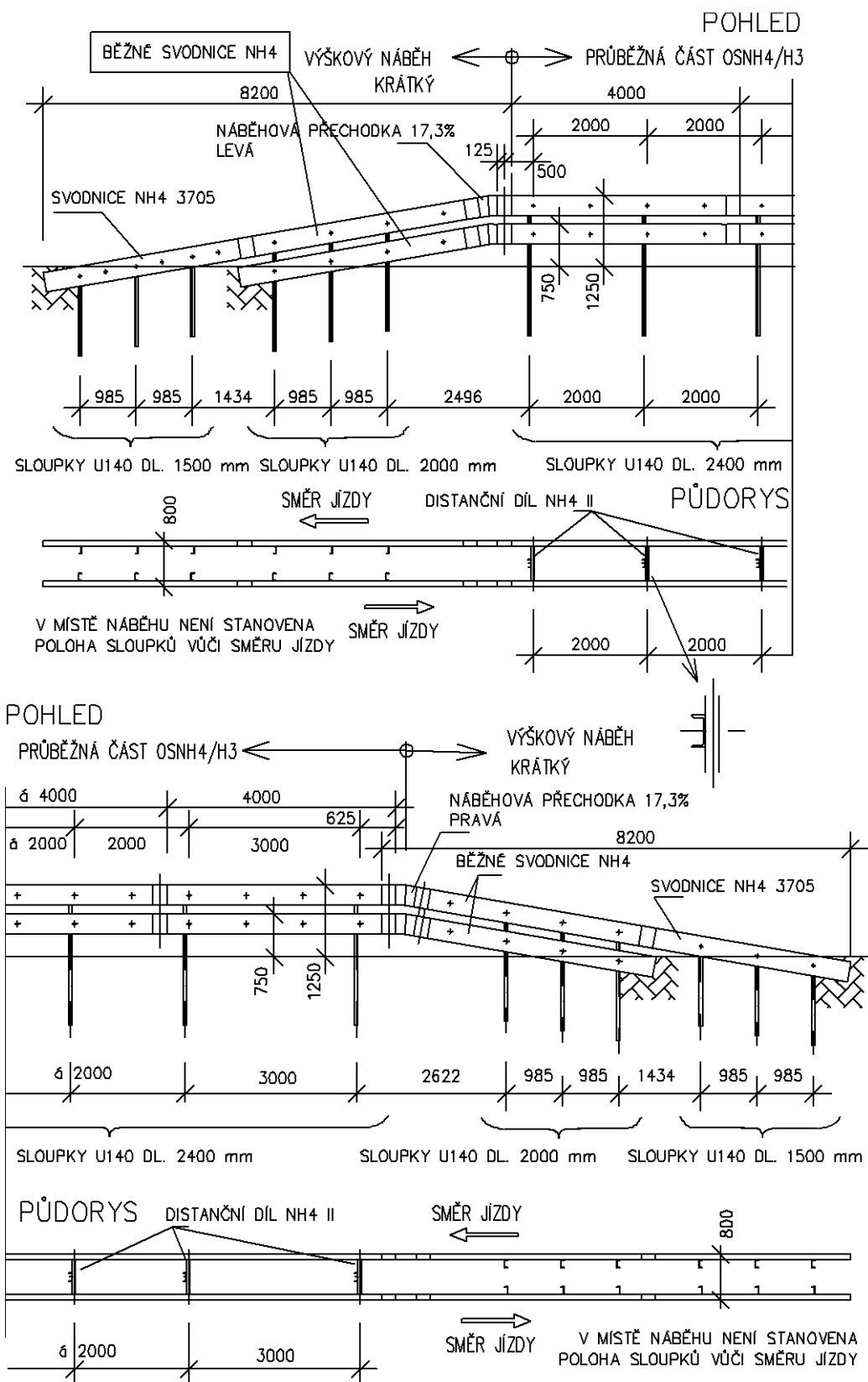
Obrázek 28 – Krátký výškový náběh svodidla OSNH4/H3
