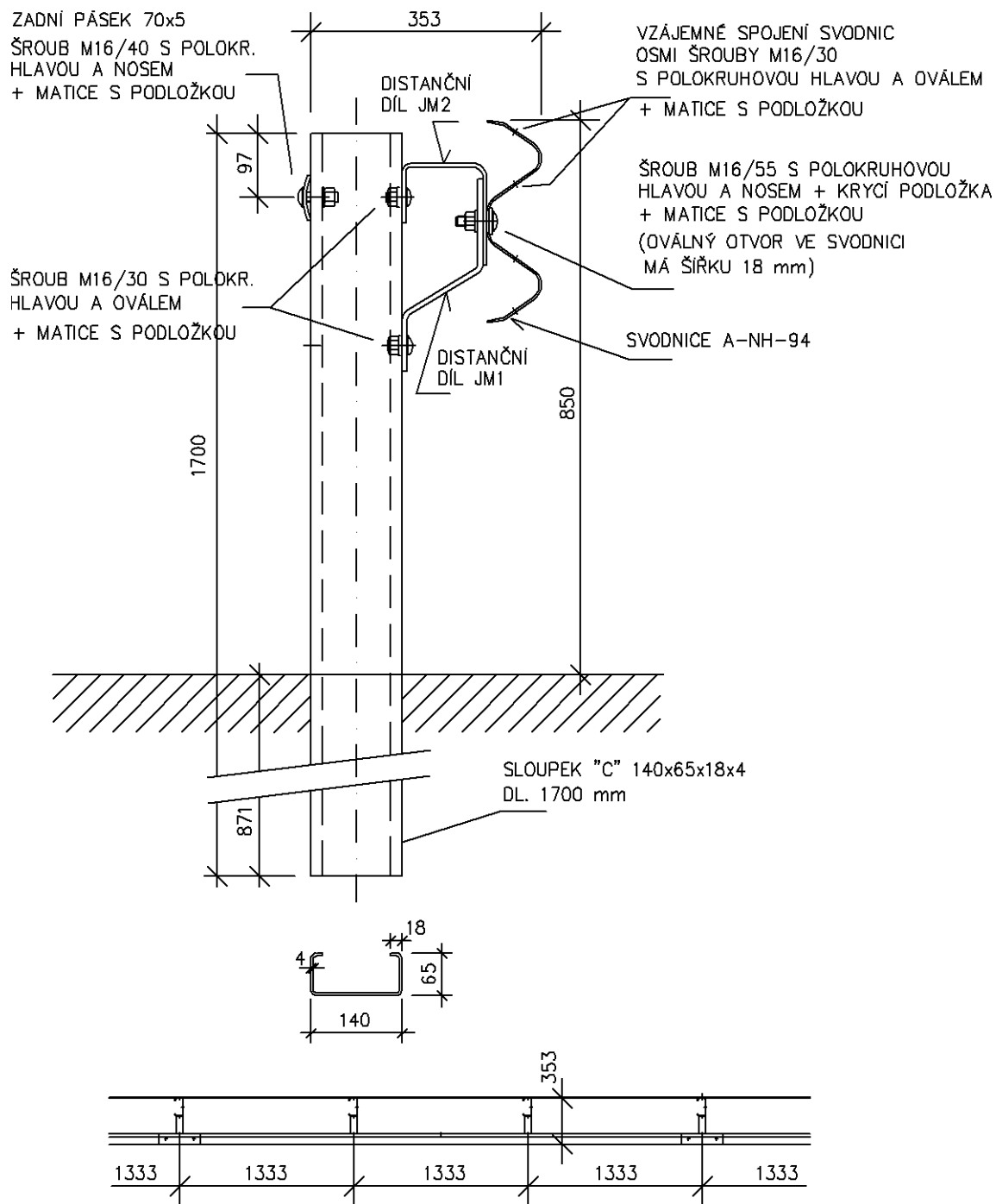
Obrázek 20 - Svodidlo J3A-1,3/H2-1
