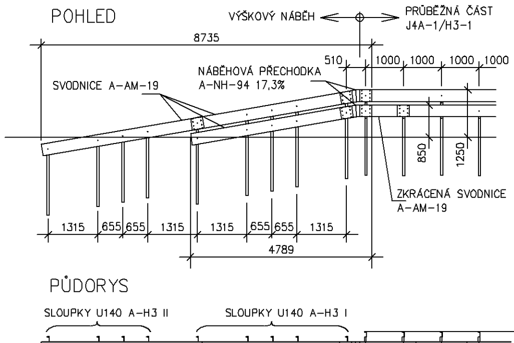
Obrázek 52 – Výškový náběh svodidla J4A-1/H3-1
