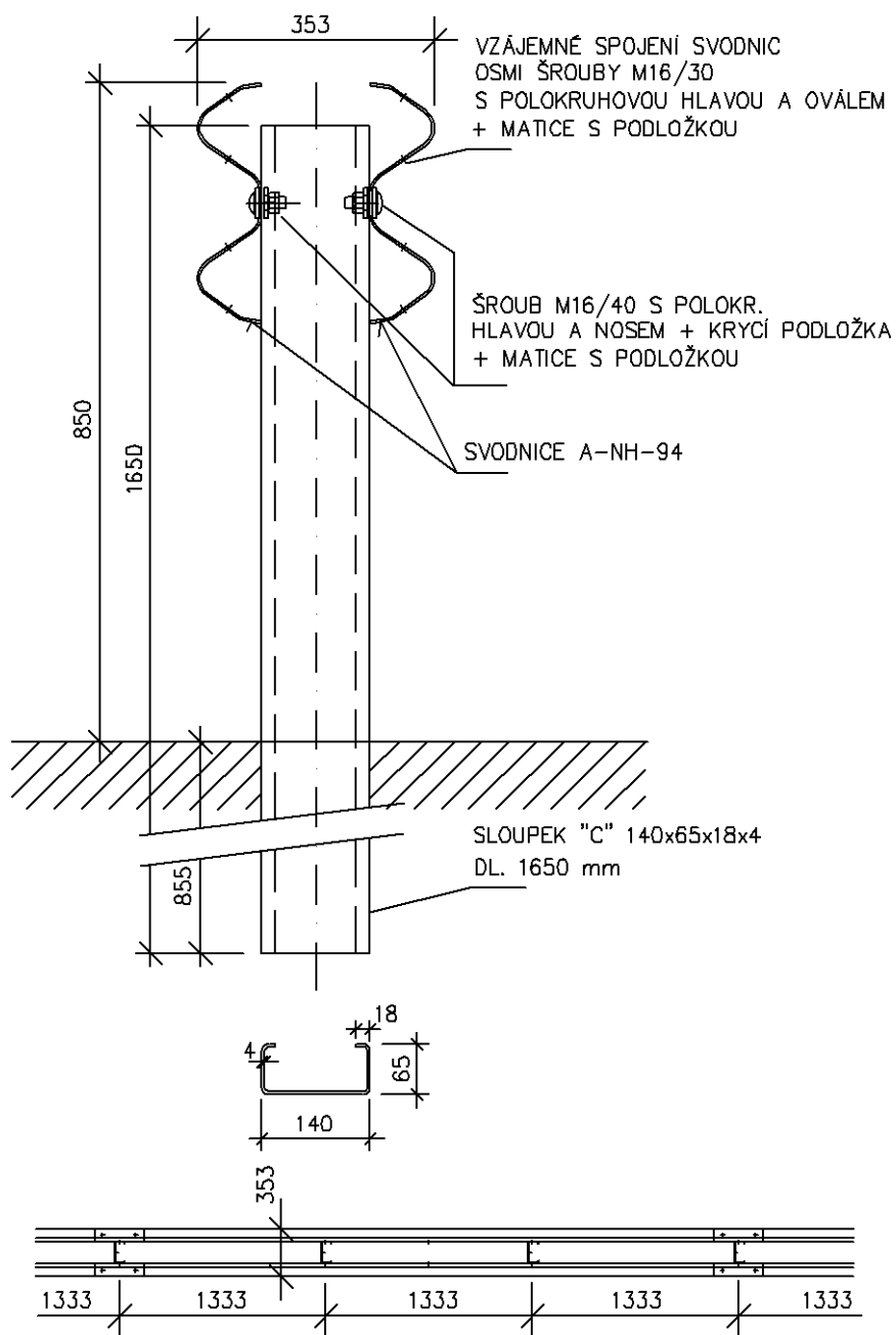
Obrázek 21 - Svodidlo 03A-1,3/H2-1
