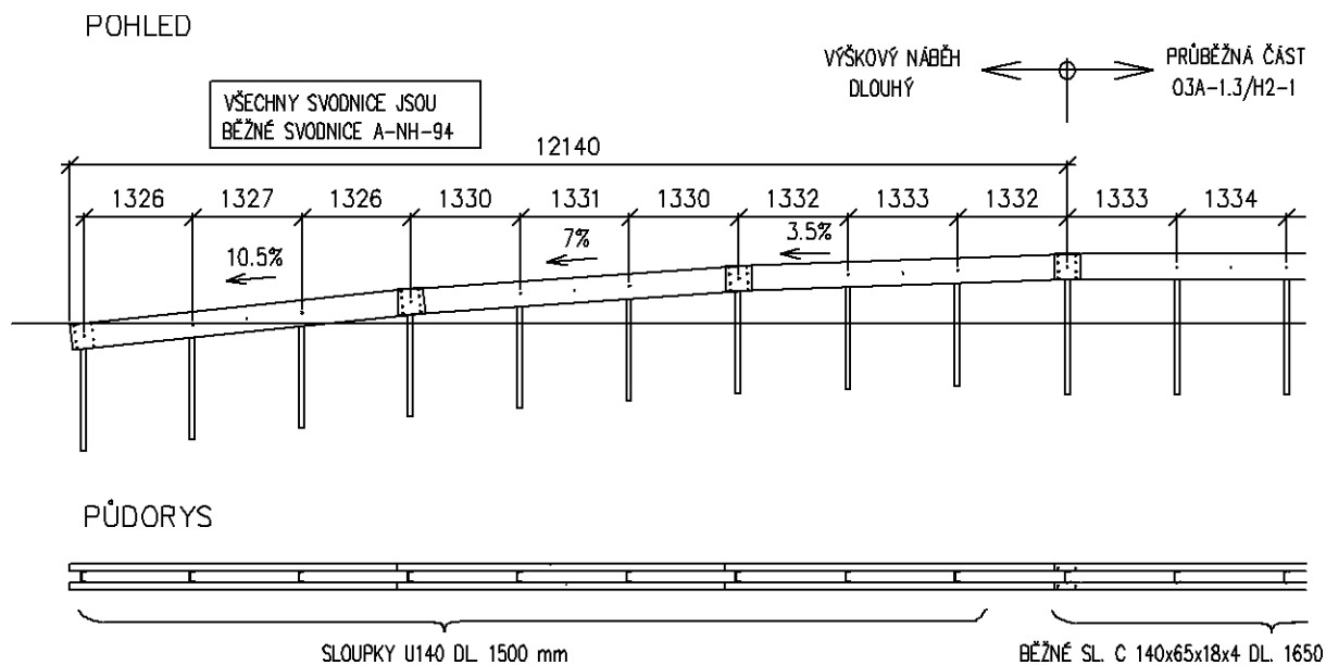
Obrázek 50 – Dlouhý výškový náběh svodidla 03A-1,3/H2-1
