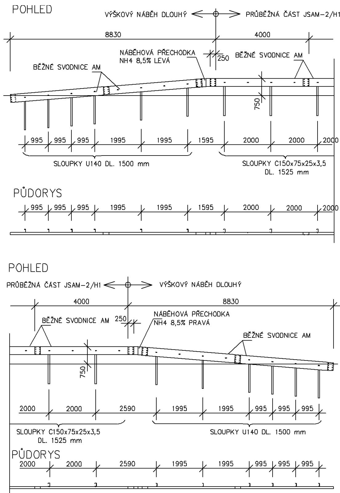
Obrázek 31 – Dlouhý výškový náběh svodidla JSAM-2/H1
