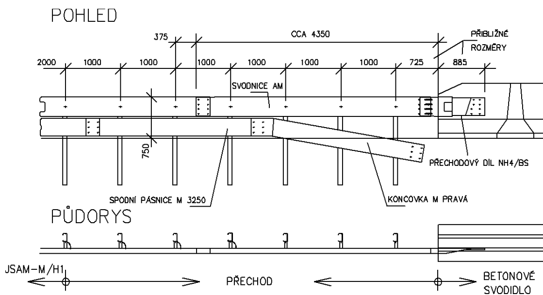
Obrázek 75 - Přejchod z JSAM-M/H1 na betonové svodidlo
