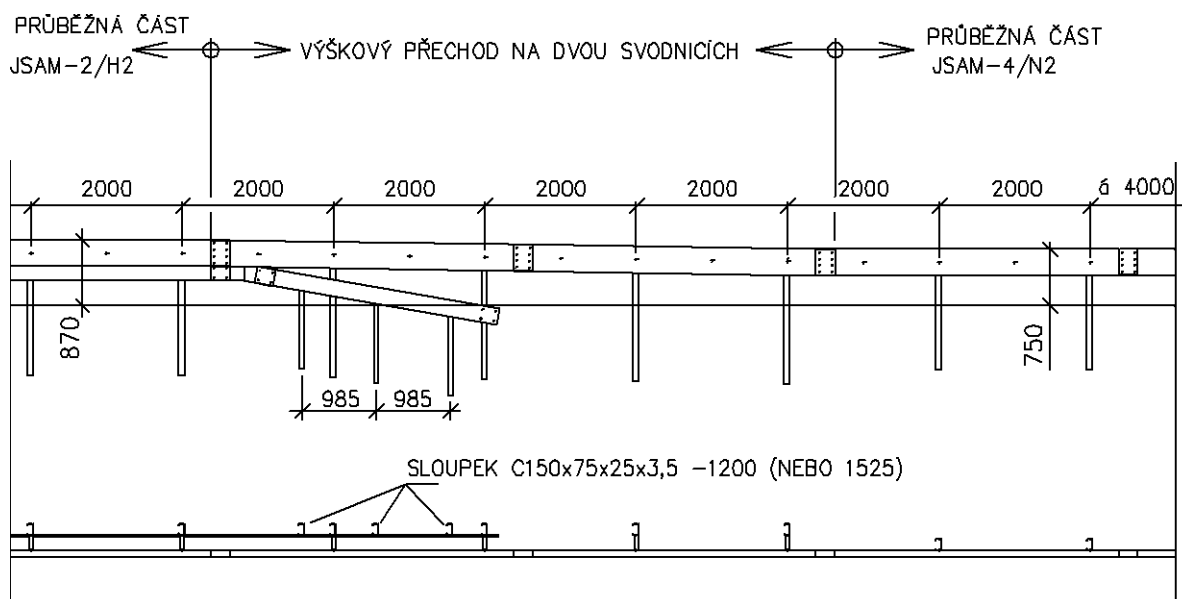
Obrázek 56 - Přejchod z JSAM-2/H2 na JSAM-4/N2
