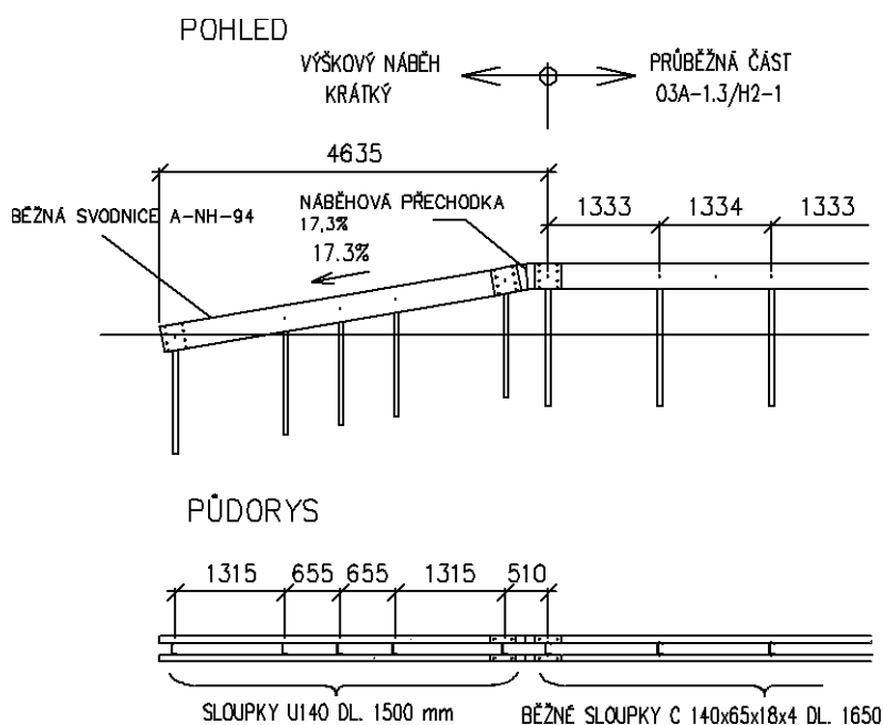
Obrázek 51 – Krátký výškový náběh svodidla 03A-1,3/H2-1
