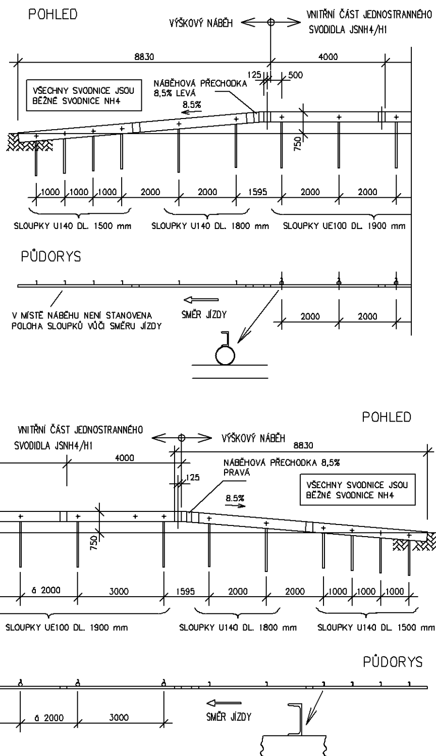
Obrázek 24 – Dlouhý výškový náběh svodidla JSNH4/H1
