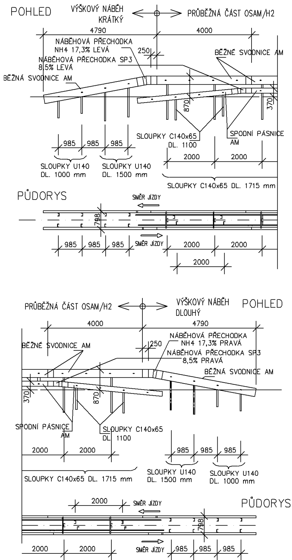
Obrázek 40 – Krátký výškový náběh svodidla OSAM/H2
