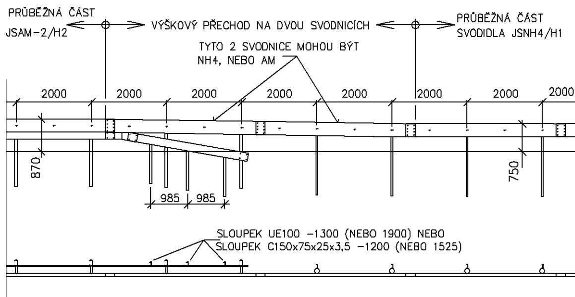
Obrázek 55 - Přejchod z JSAM-2/H2 na JSNH4/H1
