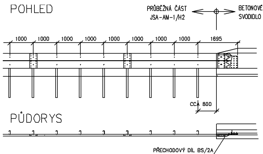
Obrázek 79 – Přejchod JSA-AM-1/H2 na betonové svodidlo
