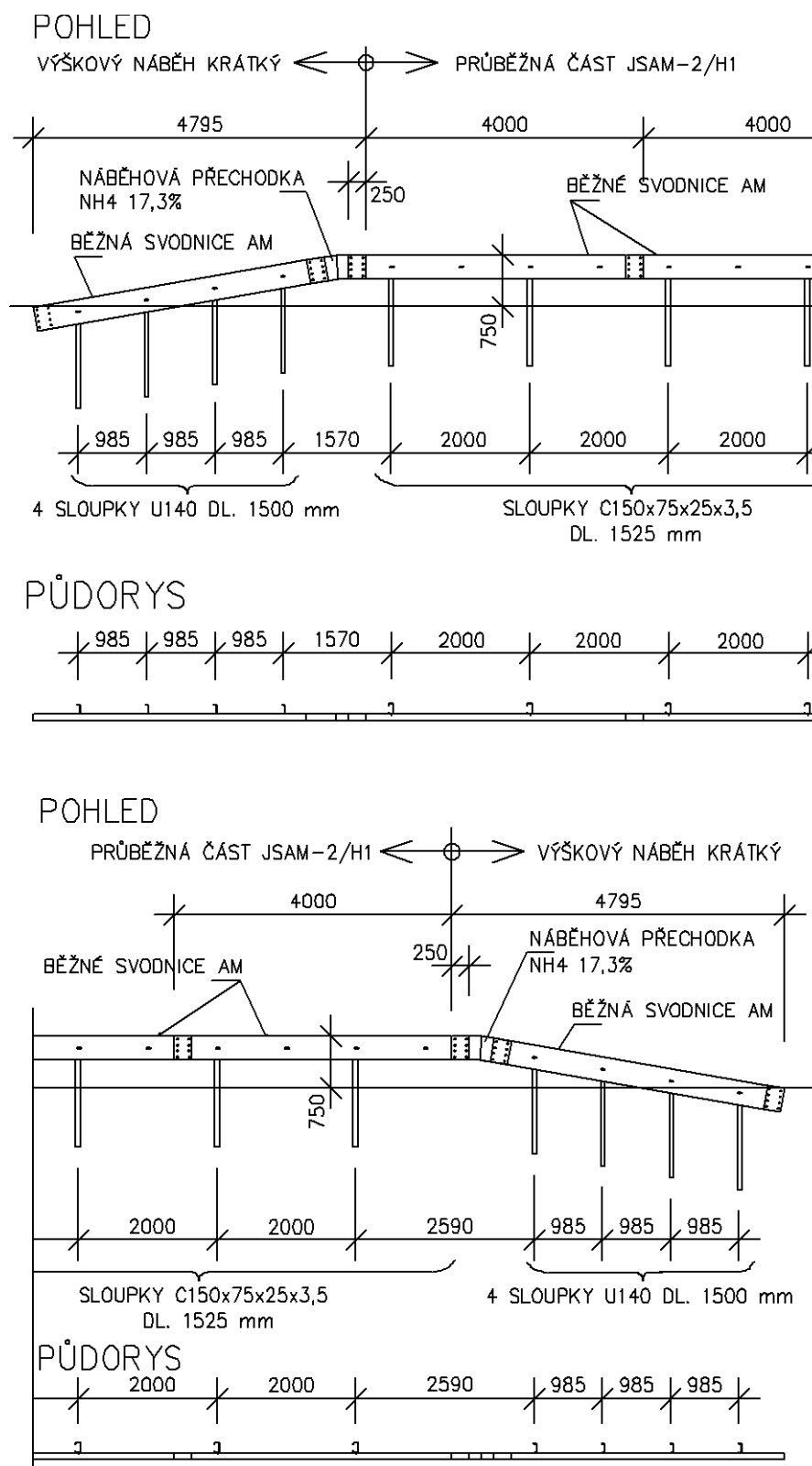
Obrázek 32 – Krátký výškový náběh svodidla JSAM-2/H1
