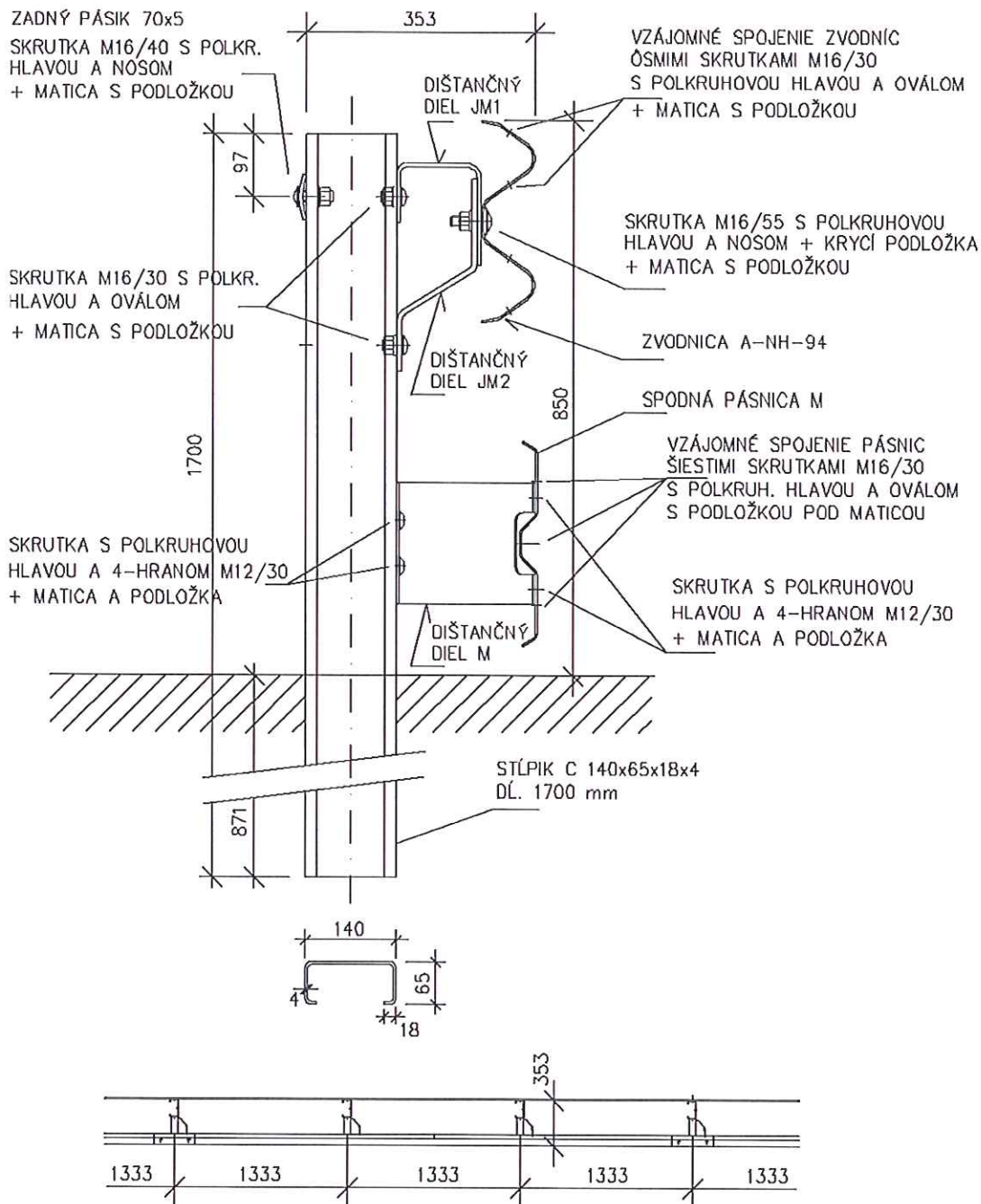
Obrázok 83 - Zvodidlo J3A-1,3M/H2-1, (v mm)
