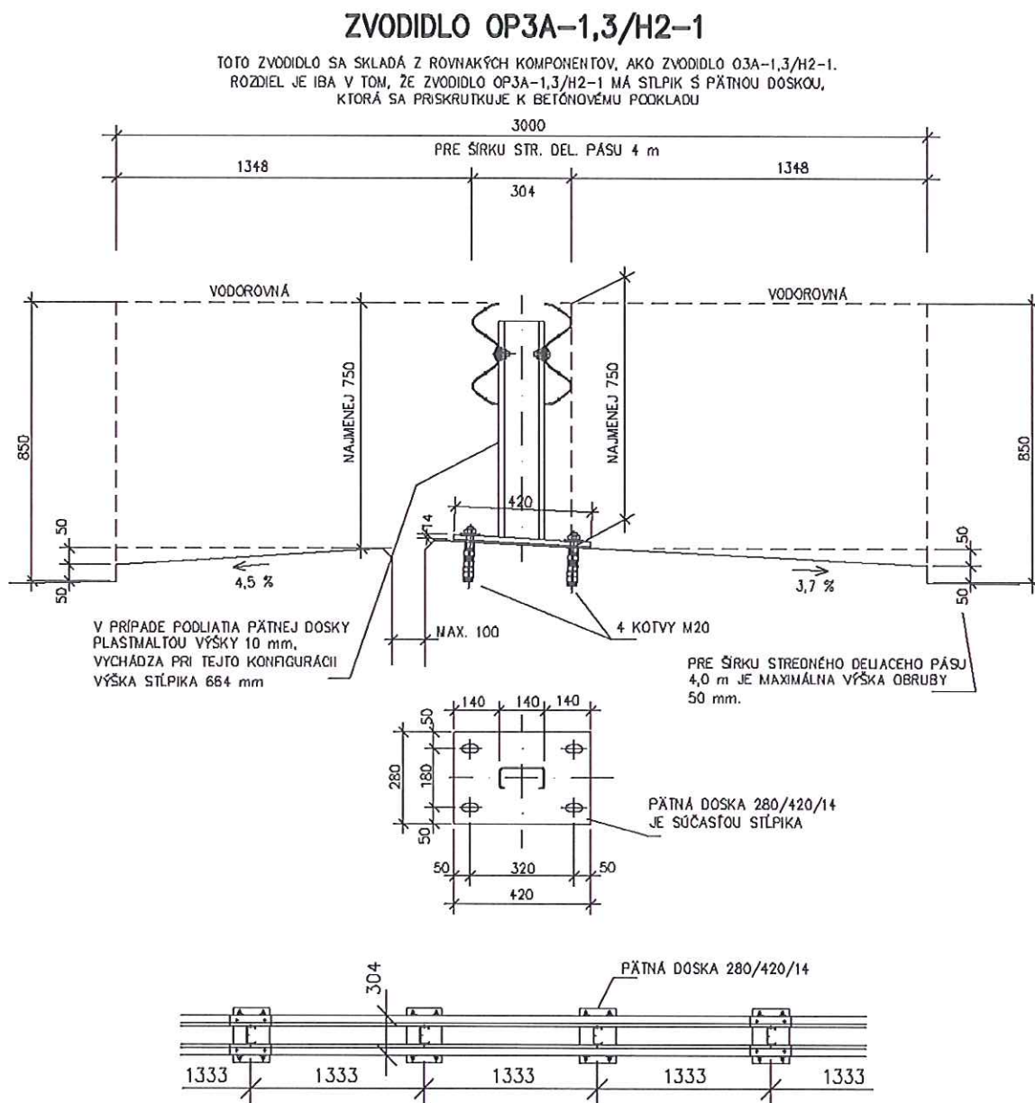
Obrázok 86 - Zvodidlo OP3A-1,3/H2-1, (v mm)
