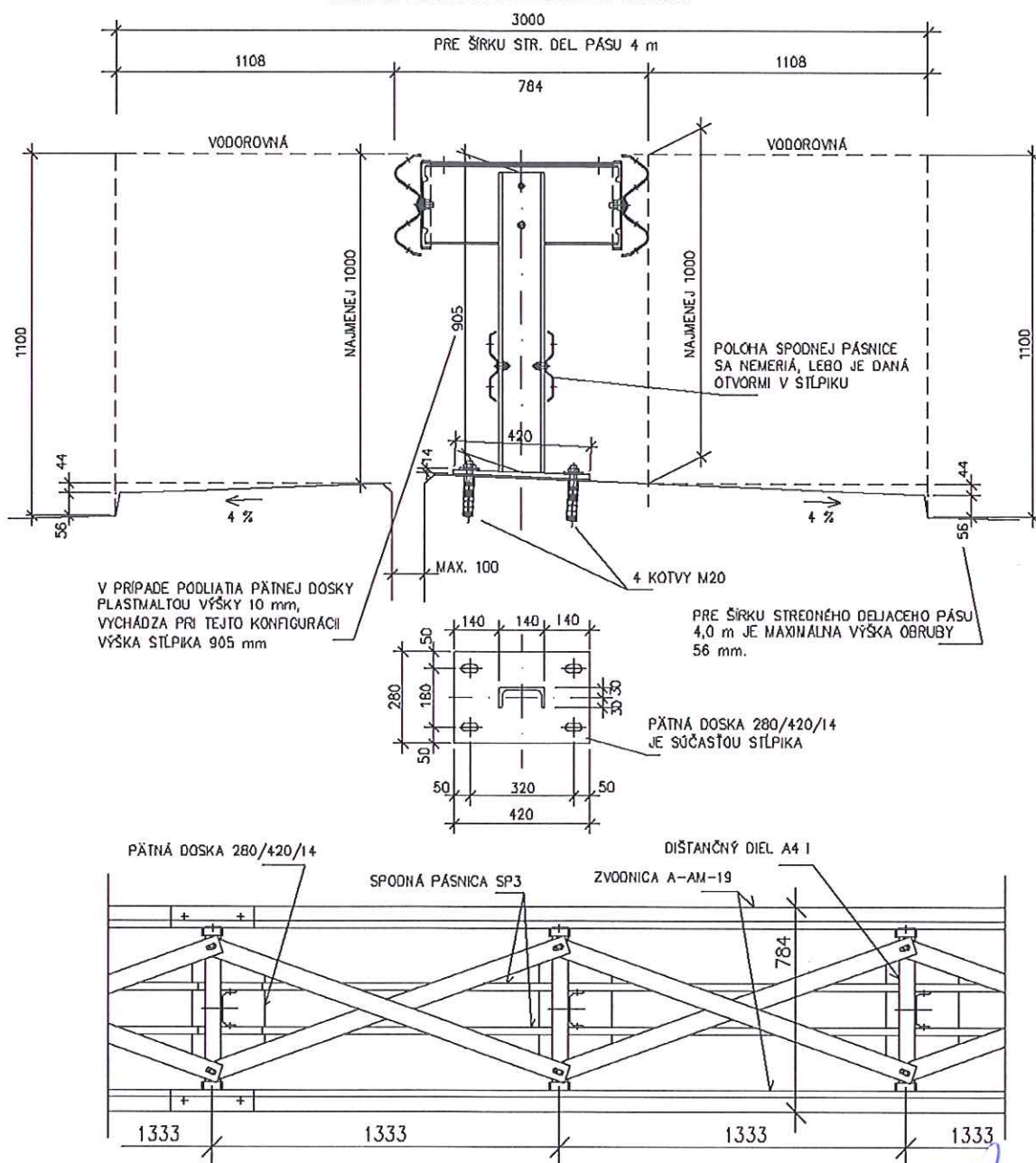
Obrázok 87 - Zvodidlo OP4A-1,3/H3-1, (v mm)
