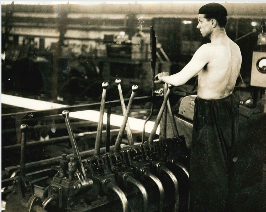
Obsluha peci pro ohřev kruhových sochorů
